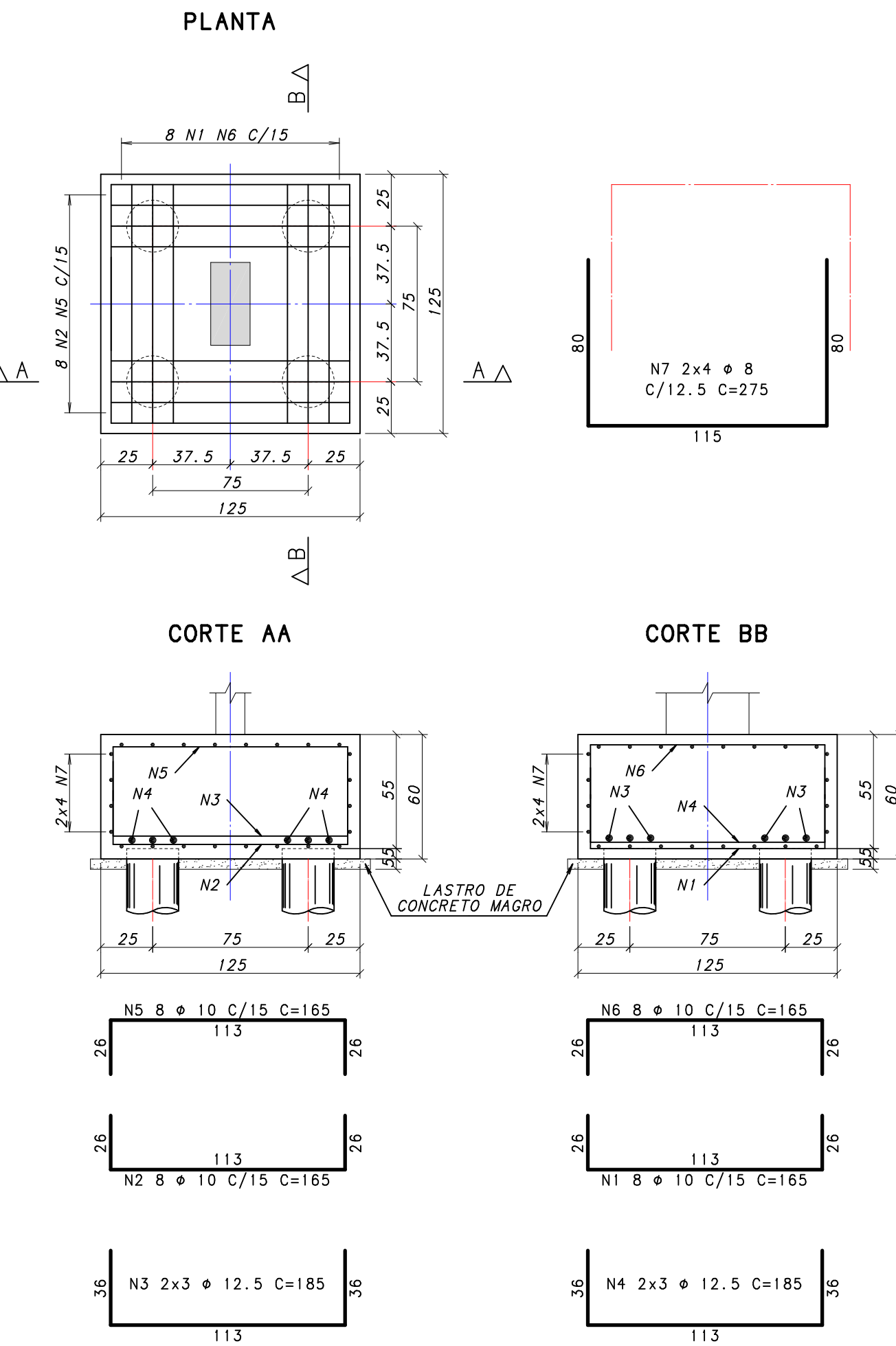
B3 125x125 h=60 Escala 1:25
