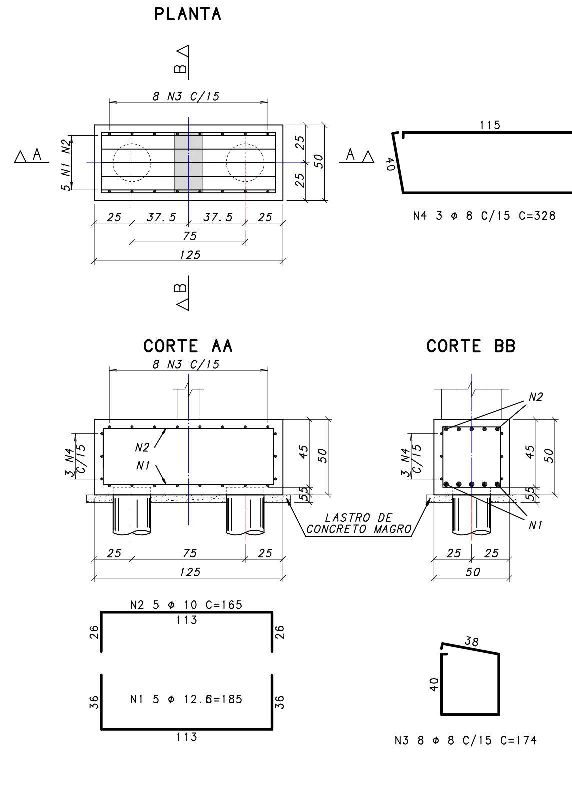
B2 125x50 h=50 Escala 1:25
