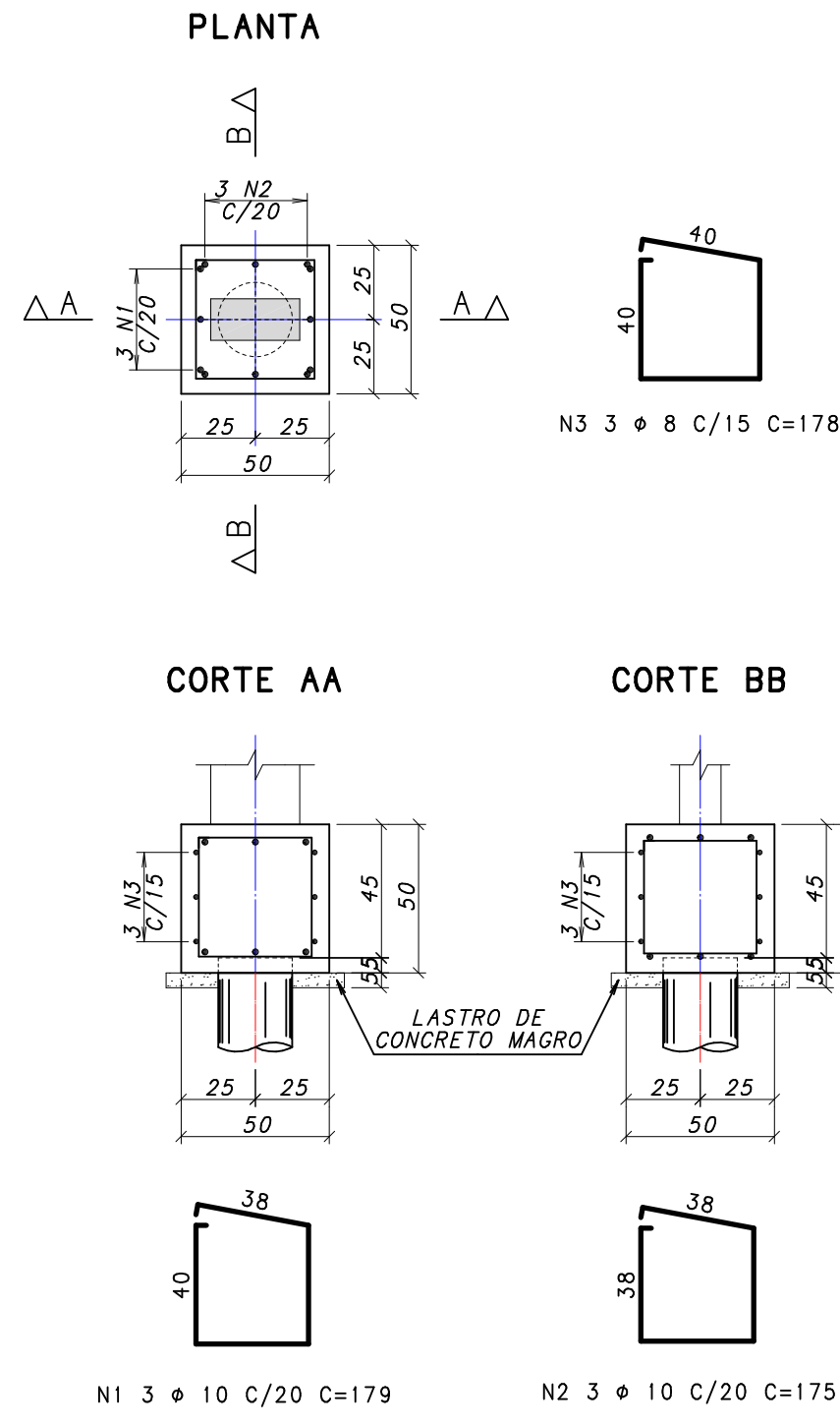
B1 50x50 h=50 Escala 1:25
